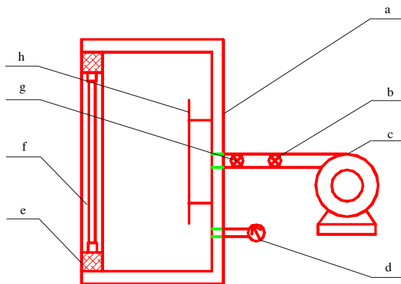
a—压力箱；b—调压系统，c—供压设备；d—压力监测仪器；e—镶嵌框； f—试件；g—流量测量装置；h—进气口挡板
